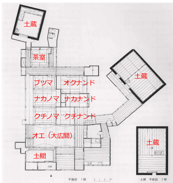
平面図（1階）
