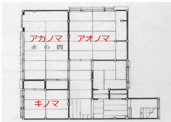
平面図（2階）
