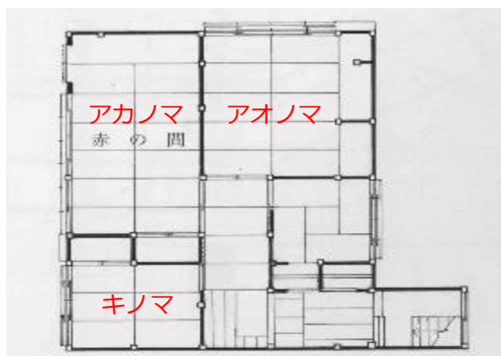
平面図（2階）
